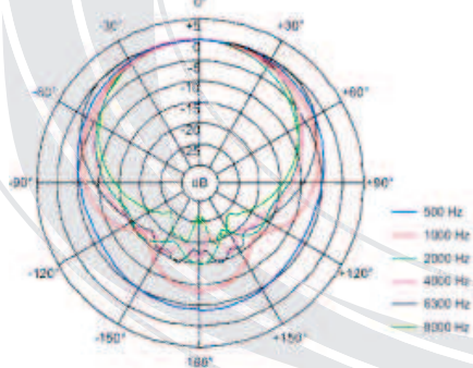
Diagramme polaire (mesuré par sinus glissant)
