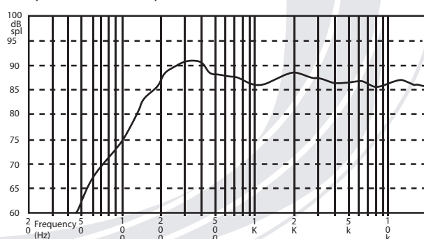
Réponse en fréquence entre 20 Hz et 20 KHz
